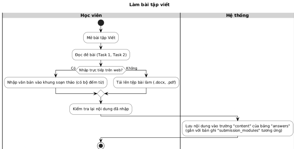
Hình 32: Hoạt động làm bài tập viết
