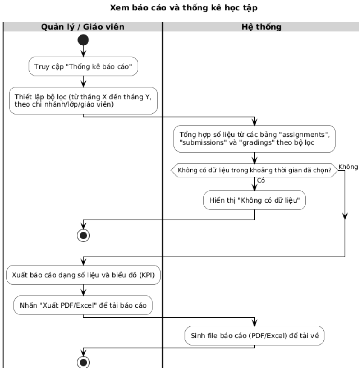
Hình 72: Hoạt động xem báo cáo và thống kê học tập
