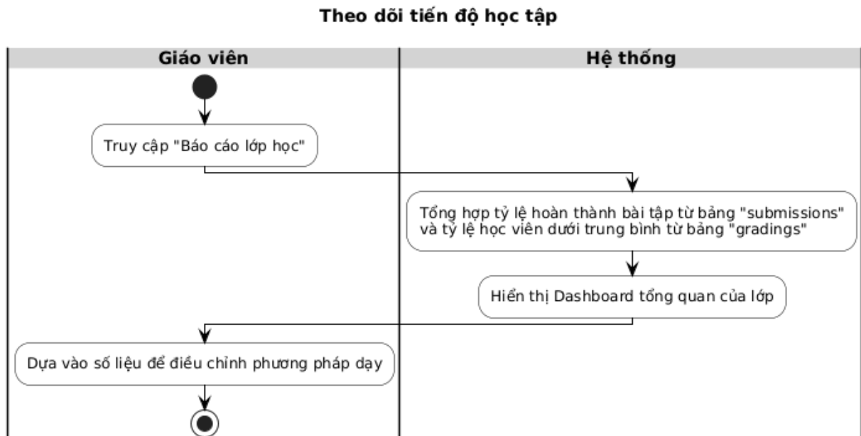
Hình 70: Hoạt động theo dõi tiến độ học tập
