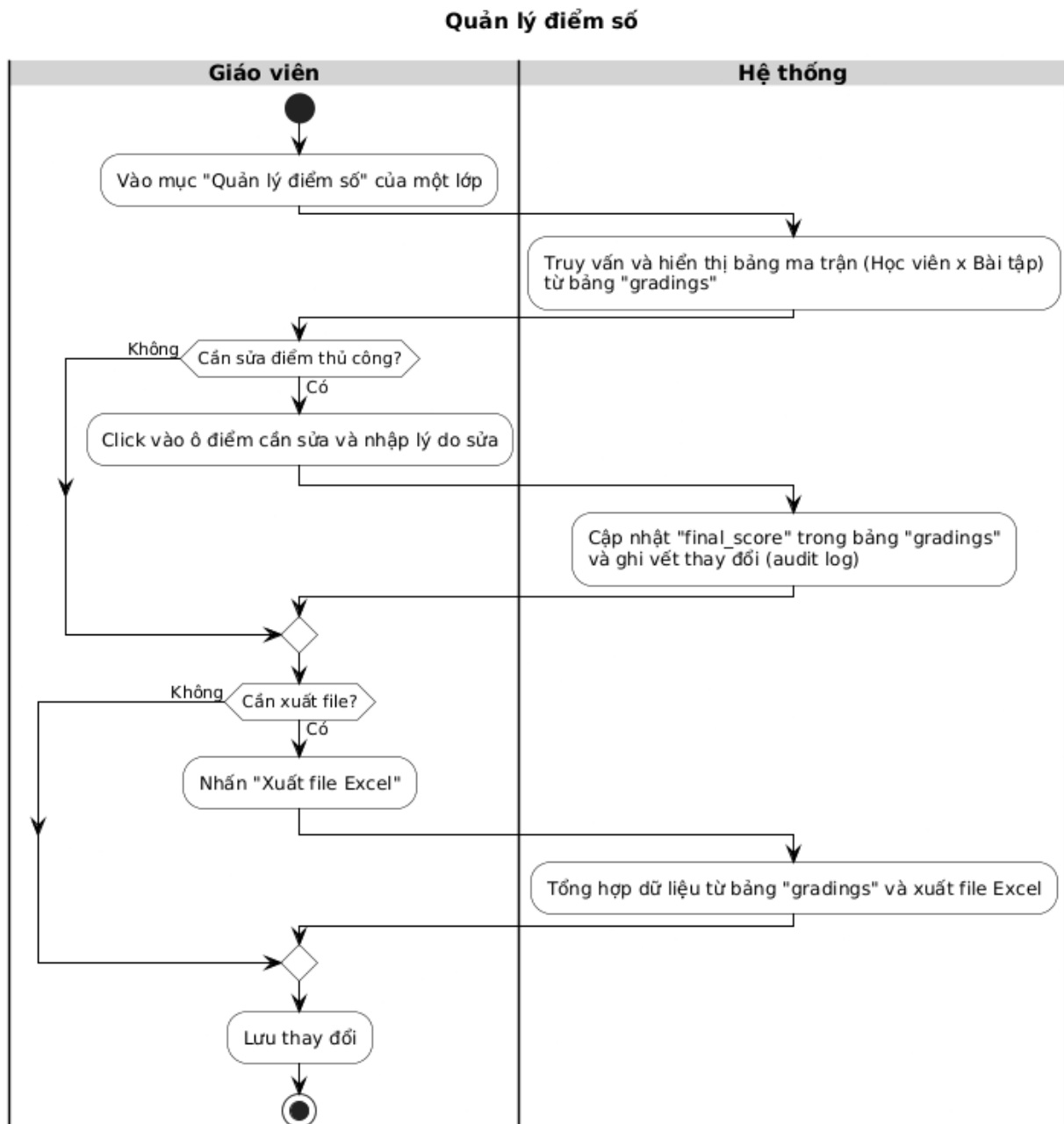
Hình 62: Hoạt động quản lý điểm số
